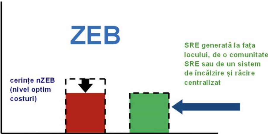
Fig. 4 Interpretarea grafică a definiției ZEB în conformitate EPBD recast (mai 2024).
